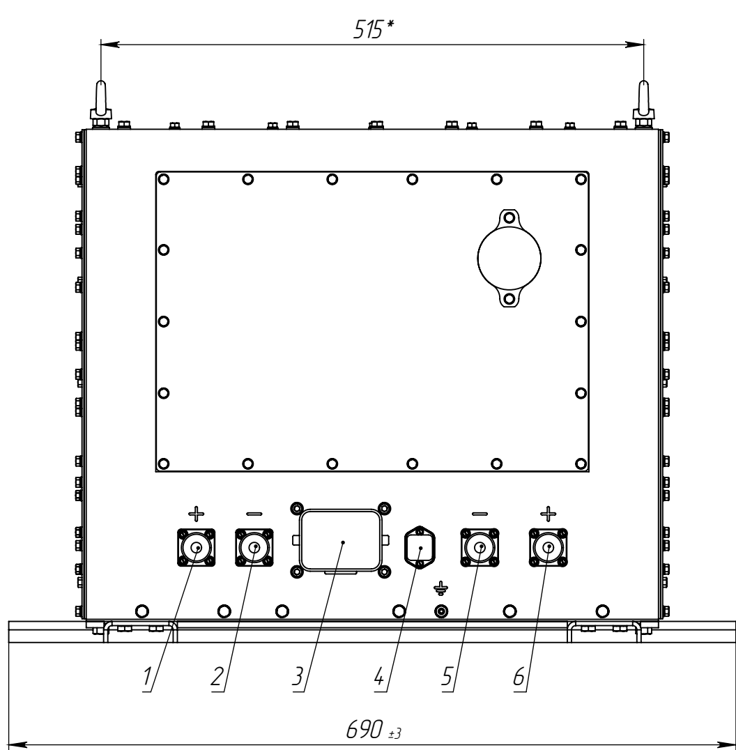
Соединительные части батарей
